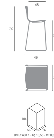
stool sled base
